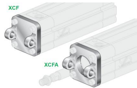
XCF - Svängfäste fram/bak ISO MP2
