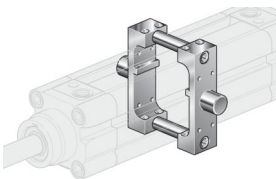
NWCIR - Midjefäste ISO MT4
