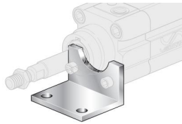
XP - Fotfäste ISO MS1
